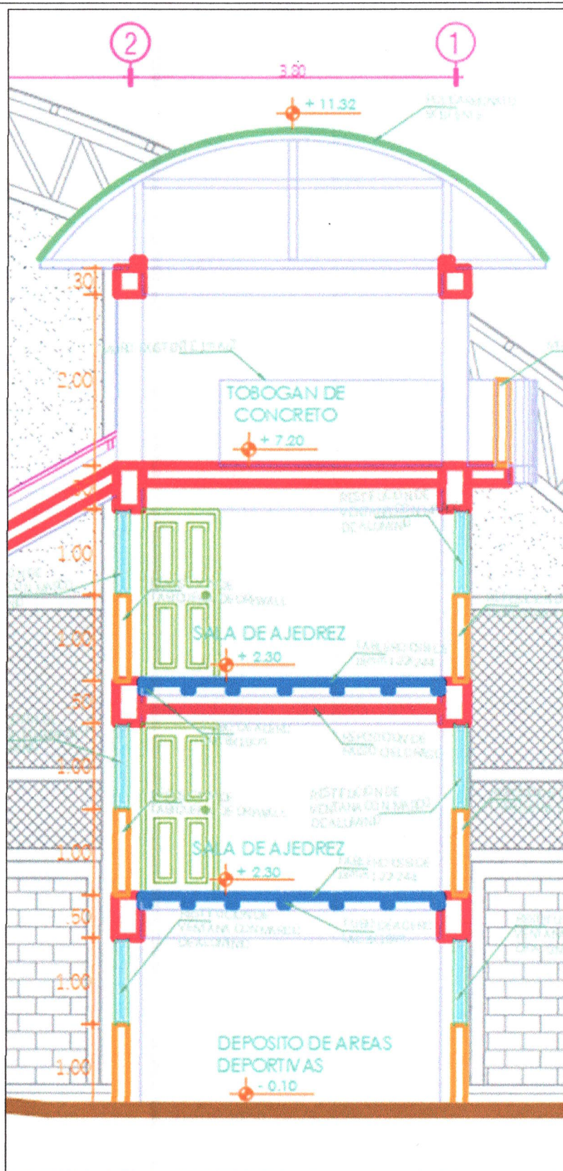
Figura N° 03: Plano de perfil de la estructura para la colocación de los muros con fibrocemento.
